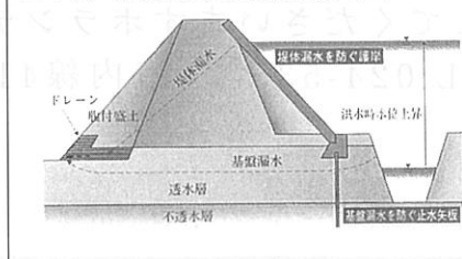
■平成の大改修堤防強化模式図
