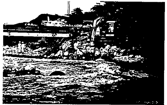
捨石投入開始
